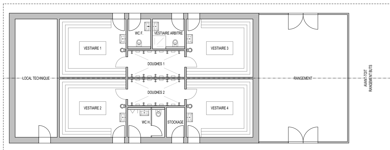
PLAN DES VESTIAIRES
